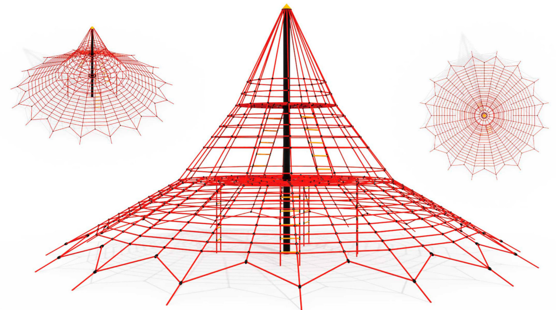
Cód: MOC-JR004 Medidas: 1100 x 1100 x 500 cm
