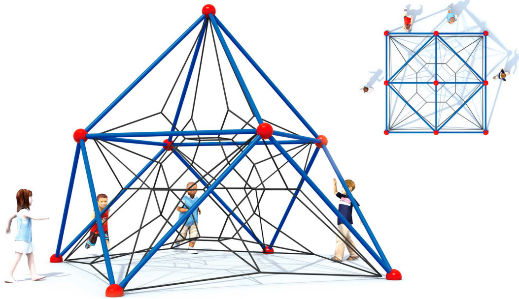
Cód: MOC-JR001 Medidas: 326 x 326 x 345 cm
