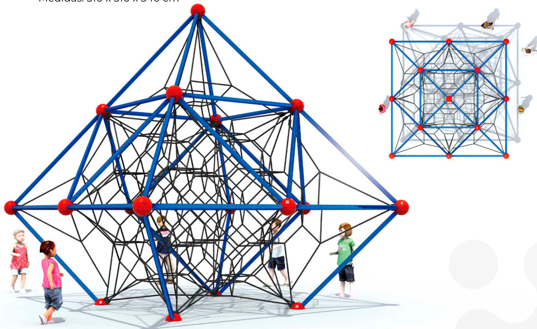
Cód: MOC-JR002 Medidas: 510 x 510 x 540 cm
