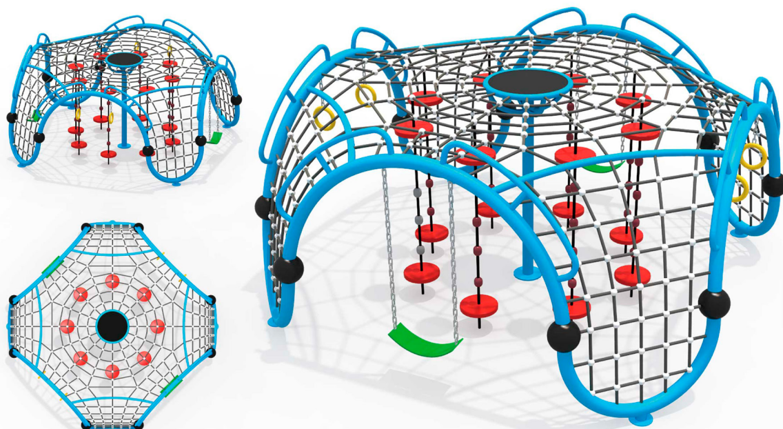
Cód: MOC-JR022 Medidas: 520 x 520 x 230 cm
