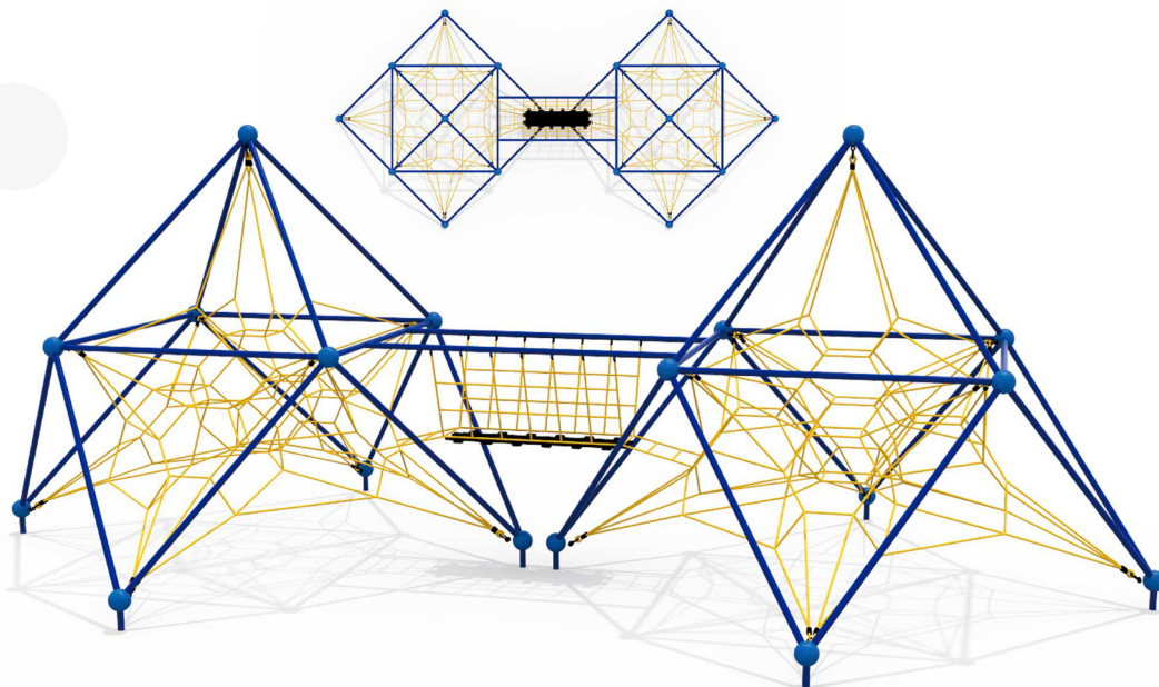
Cód: MOC-JR014 Medidas: 1050 x 500 x 390 cm
